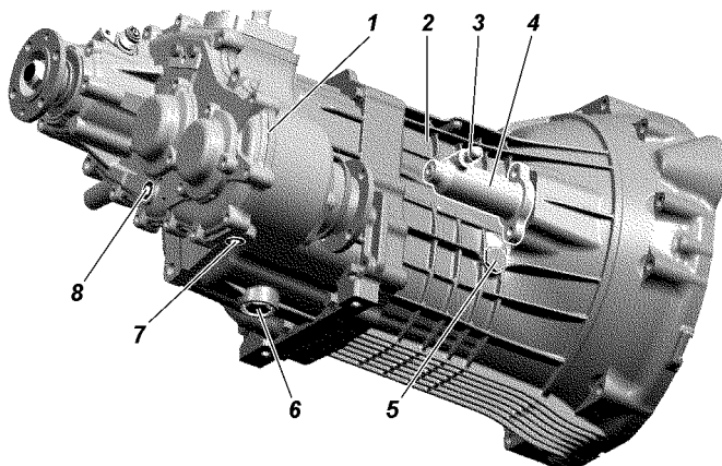
Рис. 9.23. Рабочий цилиндр выключения сцепления, пятиступенчатая коробка передач "Dymos" и раздаточная коробка:
