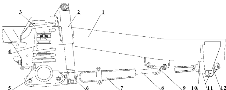
Рис. 9.29. Передняя зависимая пружинная подвеска: 1 -рама; 2 -амортизатор; 3 -пружина; 4 -буфер; 5 -мост в сборе; 6 -кронштейн амортизатора нижний; 7 -продольная штанга; 8 -штанга стабилизатора; 9 -обойма с подушкой штанги стабилизатора; 10,12 -шайба заднего конца продольной штанги; 11-втулка опорная.
