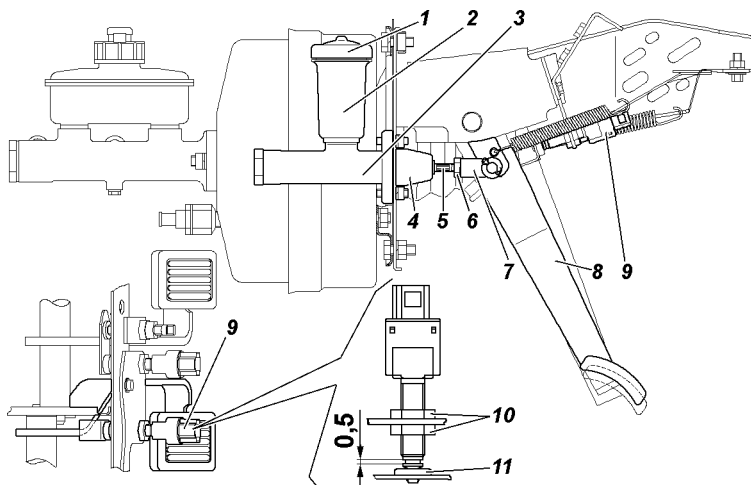
Рис. 9.21. Привод главного цилиндра выключения сцепления: 1 -крышка бачка; 2 -корпус бачка; 3 -корпус главного цилиндра; 4 -колпак защитный; 5 -толкатель; 6 -гайка; 7 -муфта толкателя; 8 -педали выключения сцепления; 9 -выключатель педали сцепления; 10 -гайки; 11 -буфер
