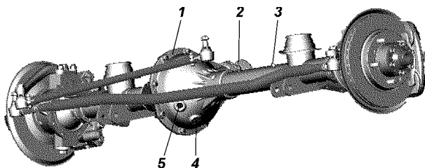
Рис. 9.26. Передний мост:
