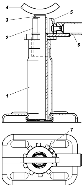
Рис. 10.2. Домкрат: 1 - шестигранник под ключ "22"
