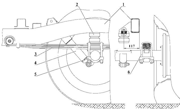
Рис. 9.30. Подвеска задняя:
