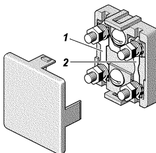
Рис. 9.50. Блок силовых плавких предохранителей: 1 - 2 -плавкие предохранители (см. таблицу)
